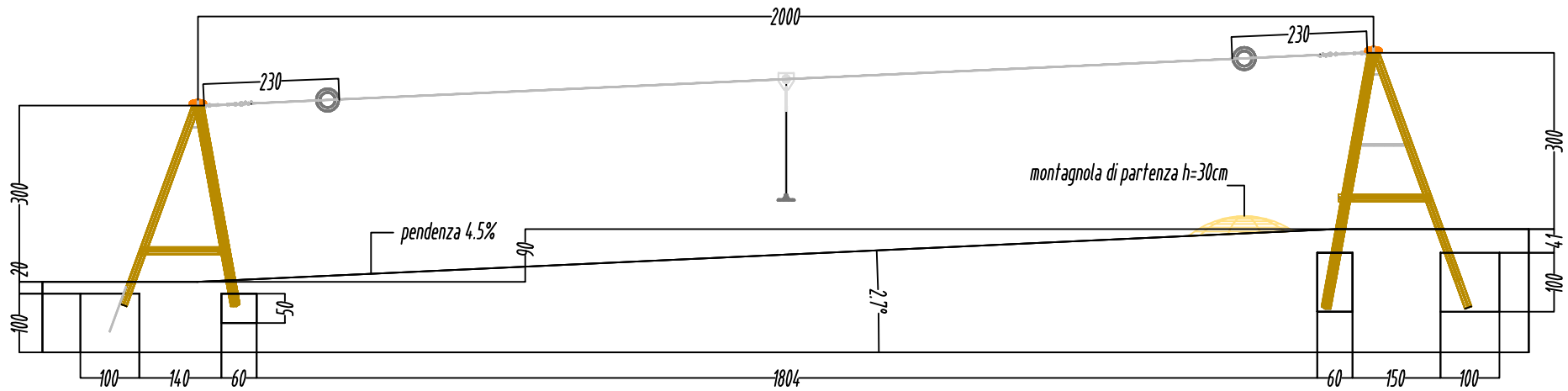
Quote, distanze e altezze per teleferica xit 101 (solo pendenza terreno)
