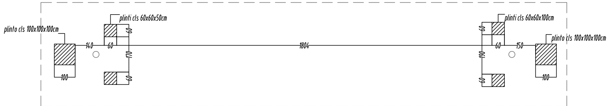
Quote, distanze e altezze per teleferica xit 101 (solo pendenza terreno)
